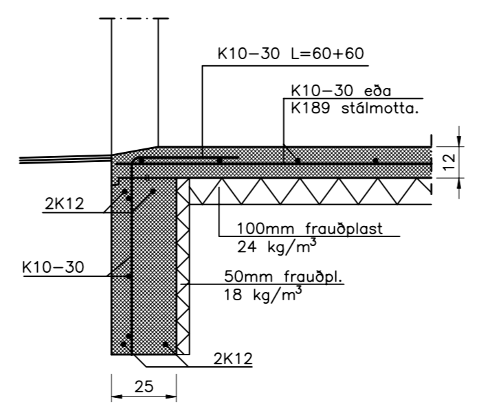
Snið 3 1:20 1701
