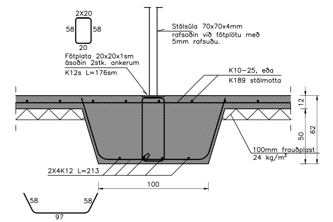
Súla S2, 1:20
