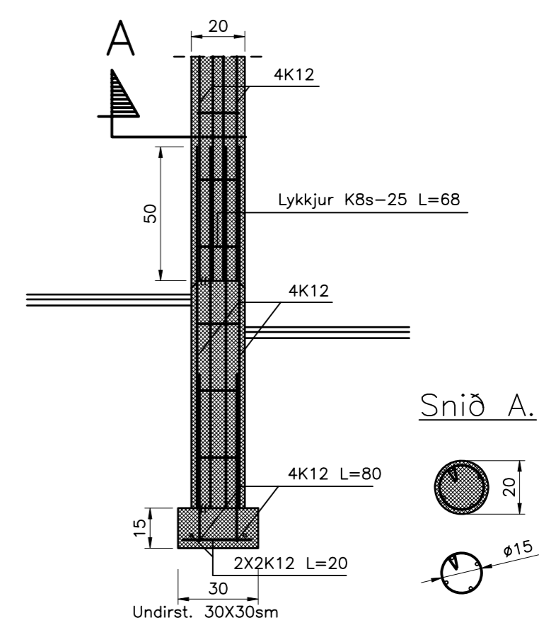
Súla S1, 1:20
