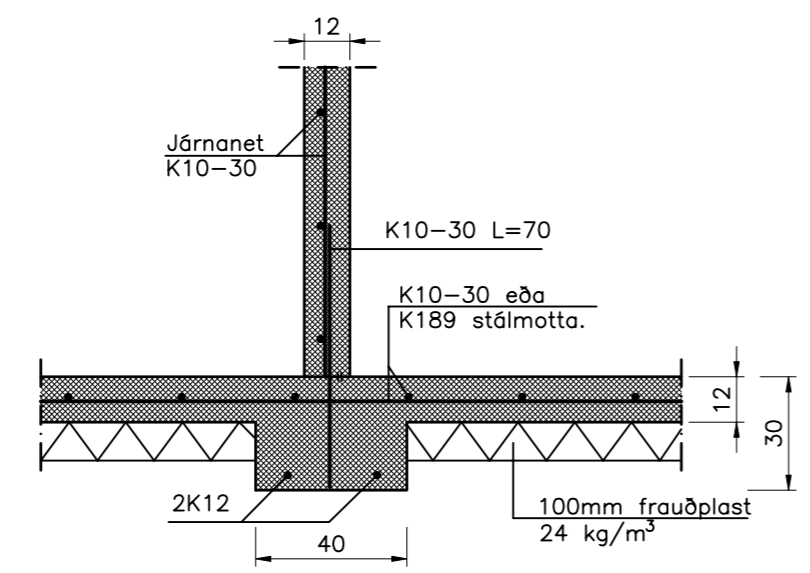
Snið 2 1:20 1701
