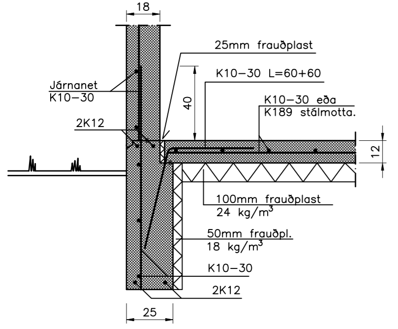
Snið 1 1:20 1701
