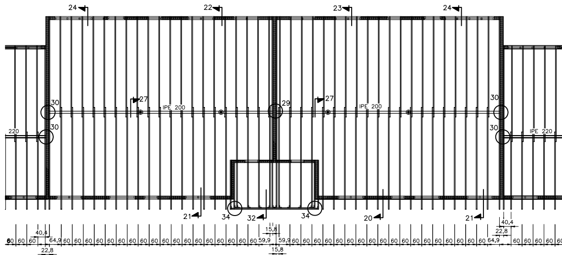
Grunnmynd þakviða hús C 1:100
