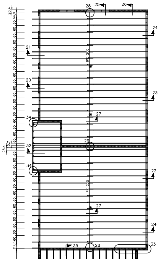
Grunnmynd þakviða hús A og E (spegilvent) 1:100
