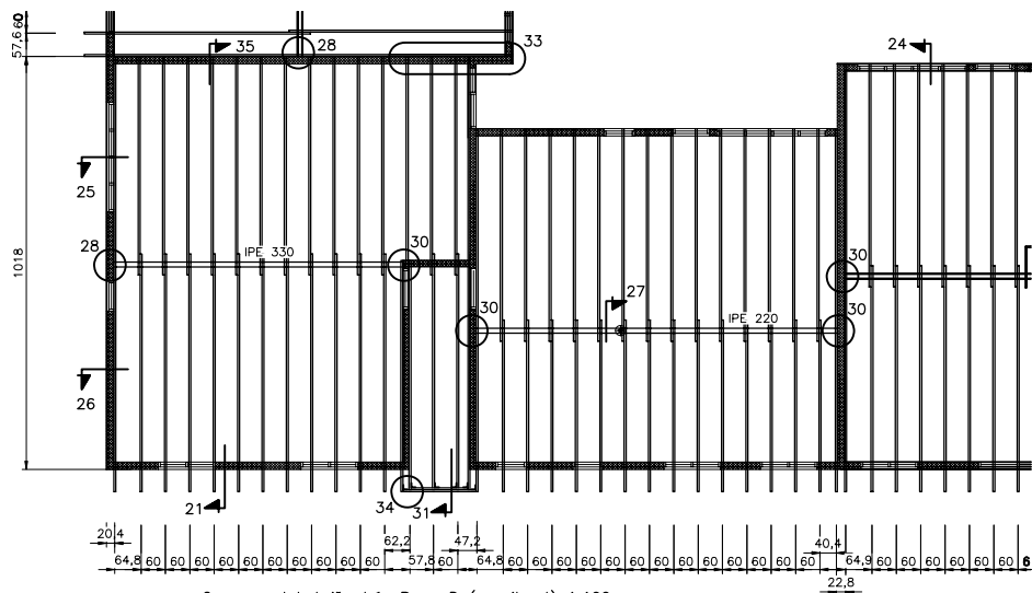
Grunnmynd þakviða hús B og D (spegilvent) 1:100
